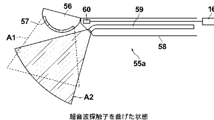
超音波探触子を曲げた状態
