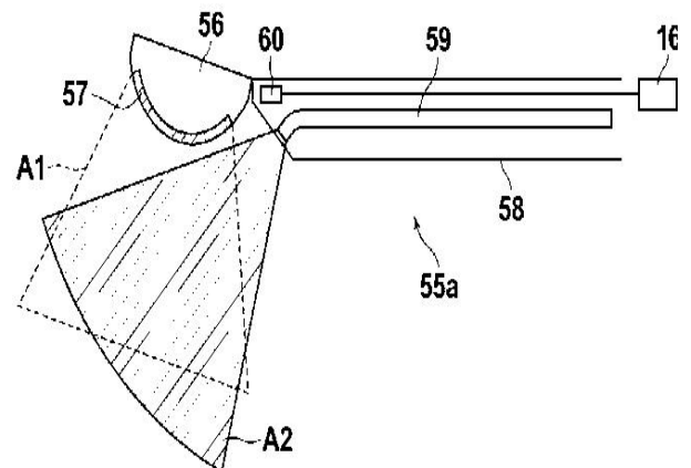
超音波探触子を曲げた状態
